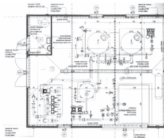
Rysunek 3. Rzut kontenera Stacji Uzdatniania Wody (1 – Hala technologiczna 58,65 m 2 , 2 – Stacja dozowania dwutlenku chloru 3,73 m 2 ).
