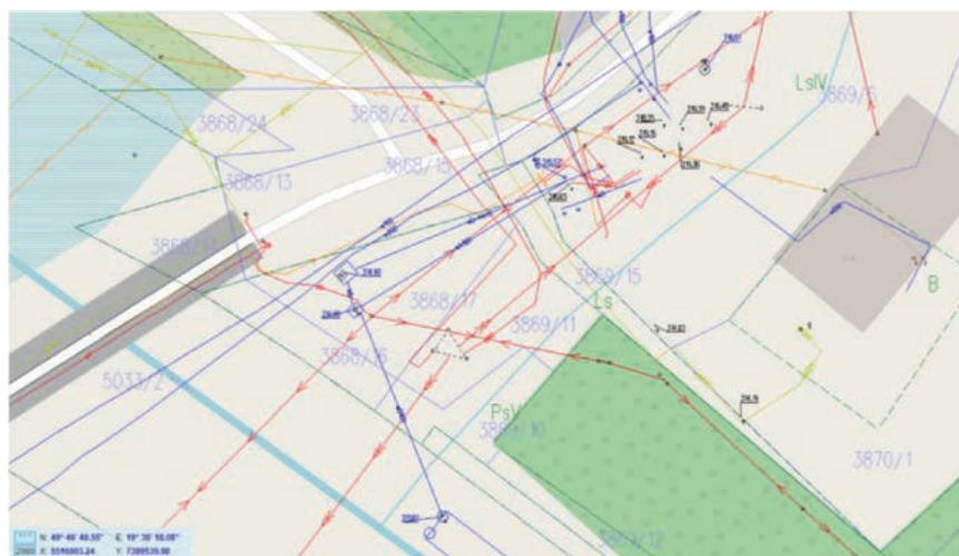
Rysunek 1. Uzbrojenie terenu przeznaczony pod inwestycję związaną z budową Stacji Uzdatniania Wody w Zembrzycach. (sieć gazowa, sieć energetyczna, sieć telekomunikacyjna, sieć światłowodowa, ciekły wodny, sieć wodociągowa, infrastruktura drogowa i mostowa, teren zagrożony powodzią)
