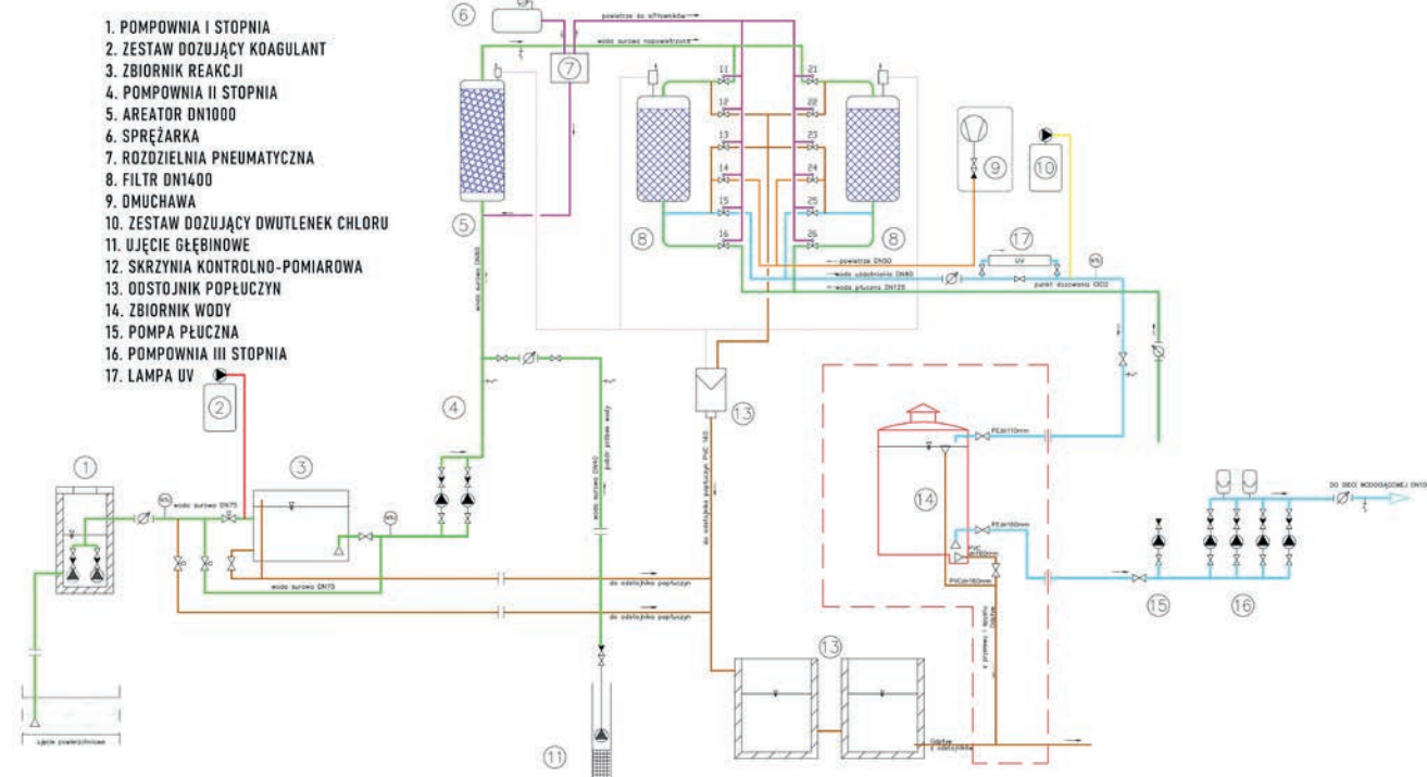
Rysunek 4. Schemat technologiczny projektowanej stacji SUW w Zembrzycach.
