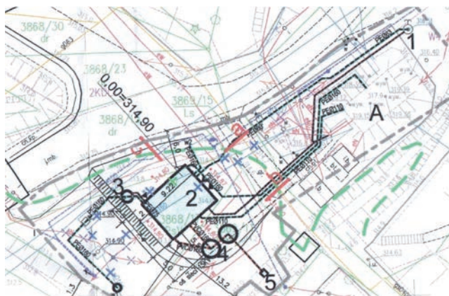
Rysunek 2. Umiejscowienie Stacji Uzdatniania Wody w Zembrzycach (1 – Studnia głębinowa, 2 – Kontenerowa SUW, 3 – Pompownia wody surowej, 4 – Odmulniki, 5 – Wylot wód popłucznych, A – Istniejący zbiornik).
